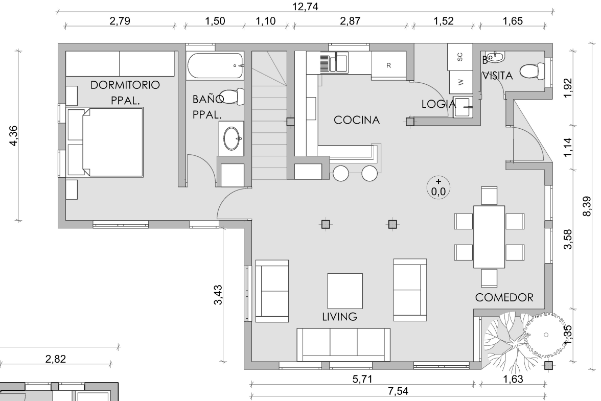
PLANTA PRIMER PISO 1:50
